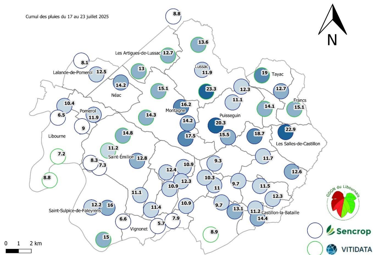
Figure 1 : Pluviométrie cumulée du 17 au 23 juillet 2025, sources : Sencrop (46 stations), Weenat (15 points)
